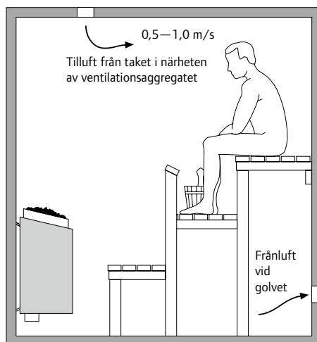
Bild 2: Ventilation av bastu
